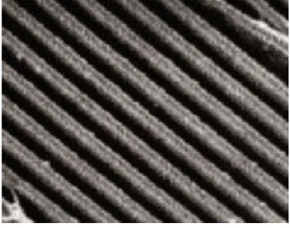
Şekil 11. Hücrenin yapışma ve yayılmasını etkileyecek mikro/nanodesenlere örnekler, (a) silikon yüzey üzerinde 80 nm eninde, 180 nm yüksekliğindeki kabartılar, (b) 7 µm genişliğinde ve 3 µm derinliğinde oluklar.
