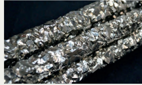
Lawrence Livermore Ulusal Laboratuvarı Zirkonyum metali
