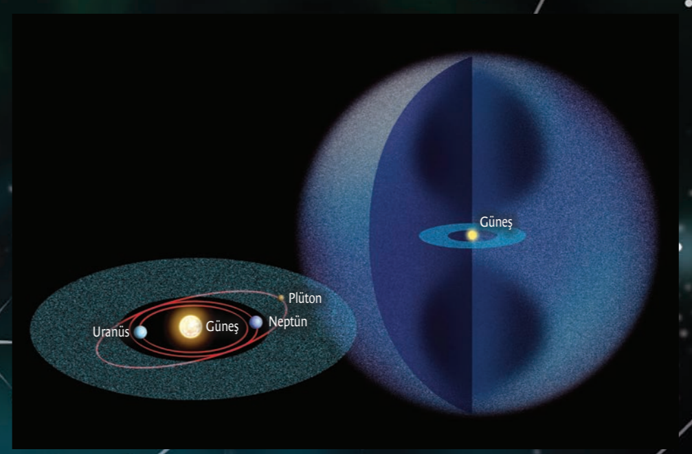
Kuiper Kuşağı (solda) ve Oort Bulutu'nun (sağda) temsili görüntüsü
