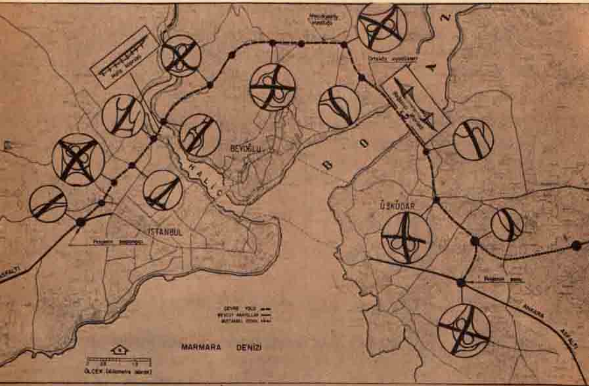
İSTANBUL ÇEVRE YOLU PLANI (HALIÇ VE BOĞAZIÇI KÖPRÜLERİ İLE KÖPRÜLÜ KAUSAKLARIN YERLERİ GÖRÜLMEKTEDİR)
